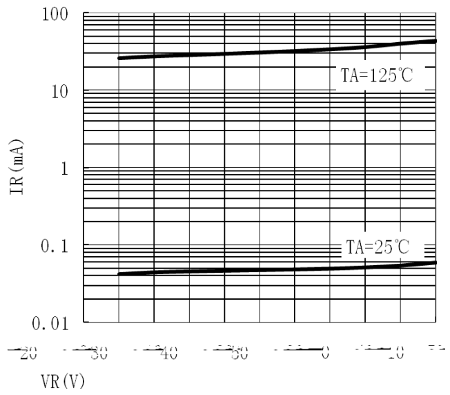
IR - VR
